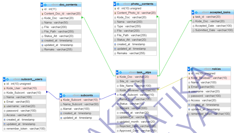
Gambar 22 Basis Data Source: Dokumentasi Pribadi
