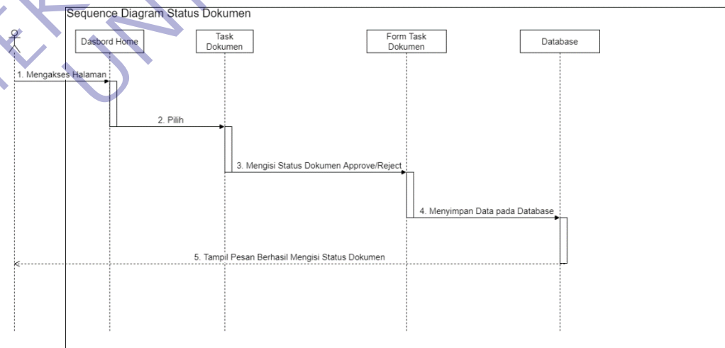
Gambar 21 Suquence Diagram Status Dokumen Source: Dokumentasi Pribadi
