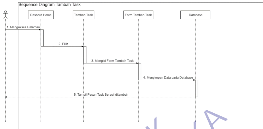
Gambar 16 Suquence Diagram Tambah Task Source: Dokumentasi Pribadi
